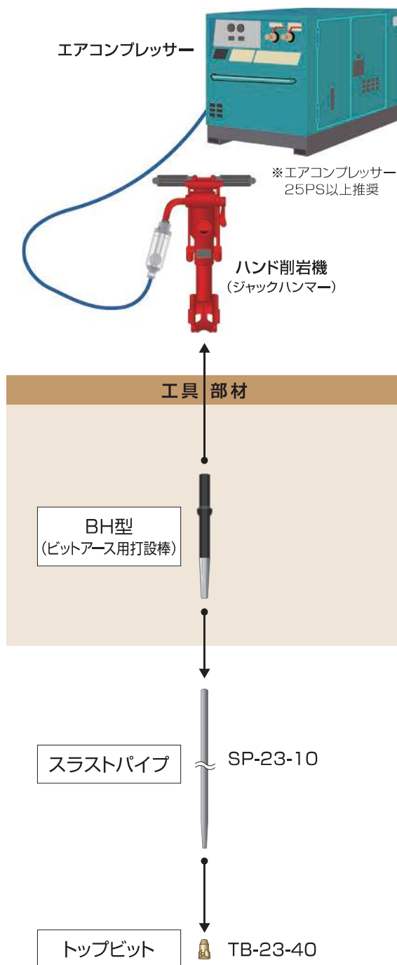
適用工具例
