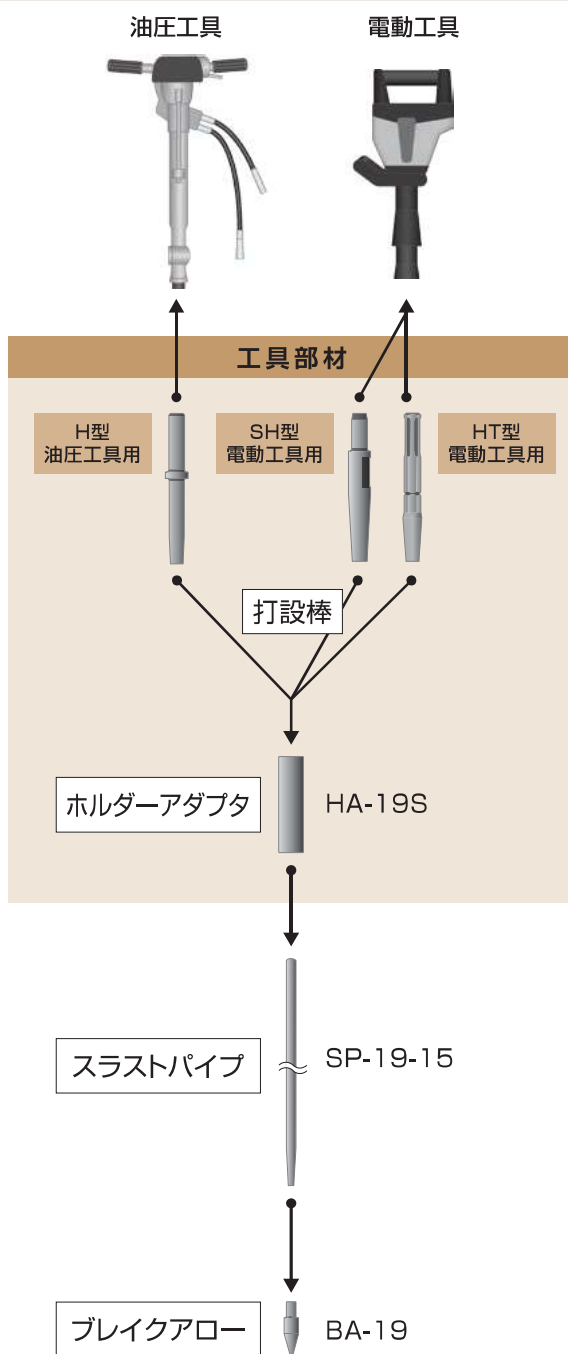
適用工具例
